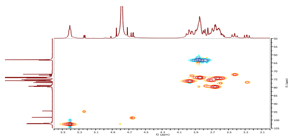
Fig 10: ^1\text{H} - ^{13}\text{C} HSQC of Sweitenia mycophylla gum
