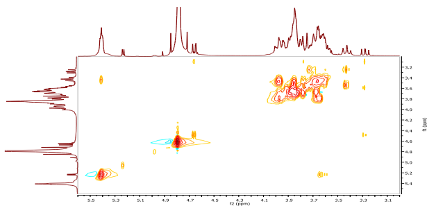
Fig 9: ^1\text{H} - ^1\text{H} TOCSY of Sweitenia mycophylla gum
