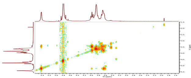
Fig 8: ^1\text{H} - ^1\text{H} COSY of Sweitenia mycophylla gum
